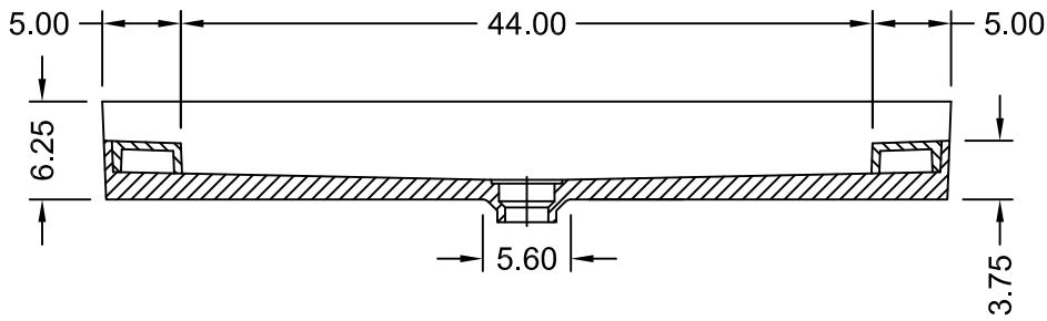
SECTION A-A
