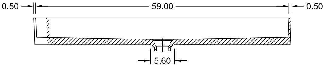
SECTION A-A
