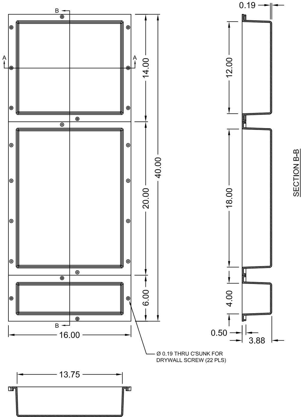
SECTION A-A
