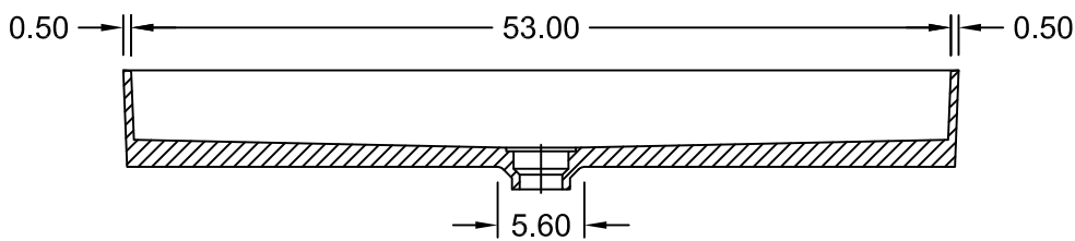
SECTION A-A
