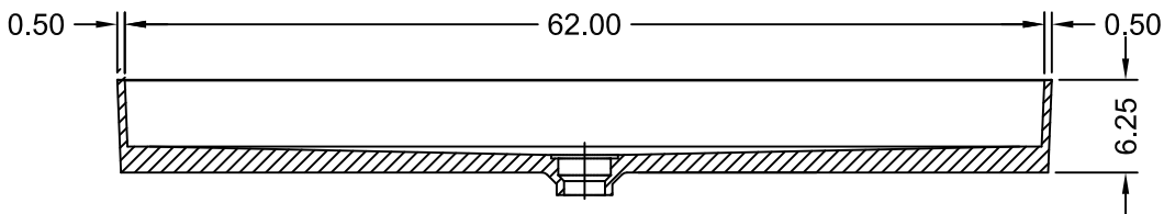
SECTION A-A
