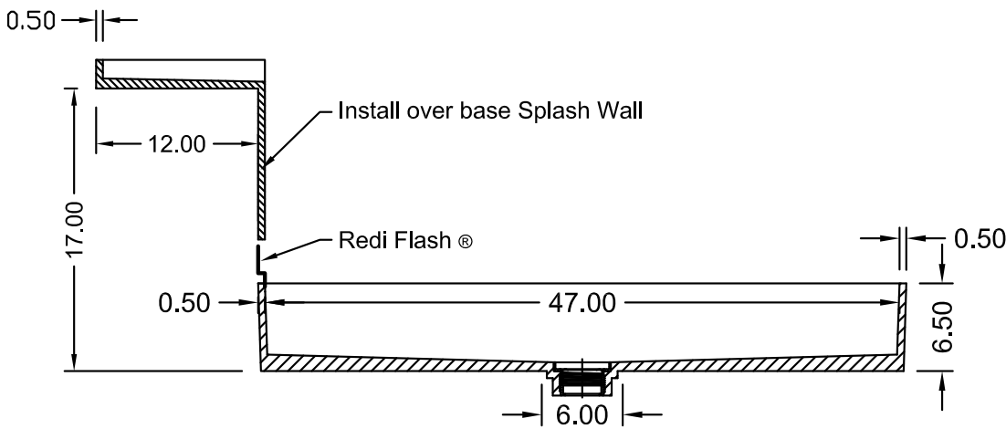
SECTION A-A
