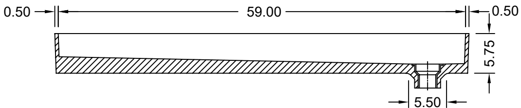
SECTION A-A
