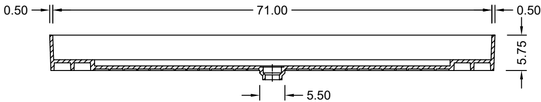
SECTION A-A
