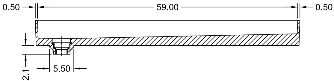
SECTION A-A
