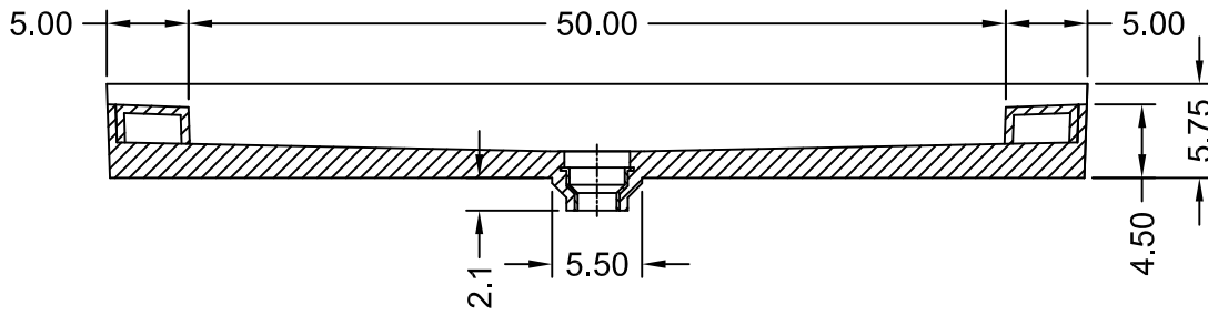
SECTION A-A
