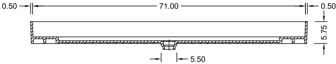
SECTION A-A
