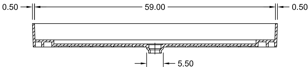
SECTION A-A
