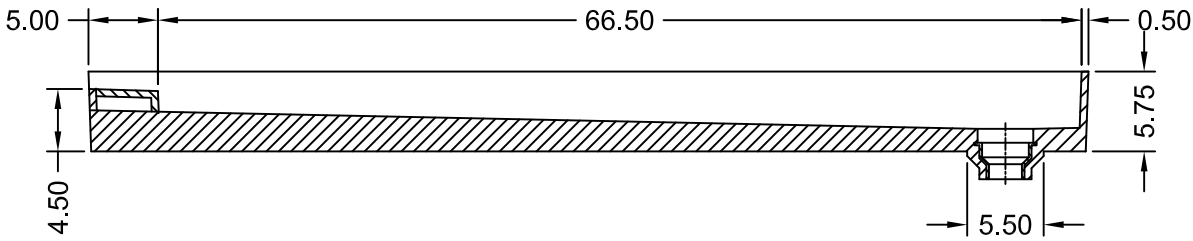
SECTION A-A
