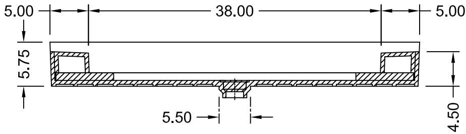
SECTION A-A
