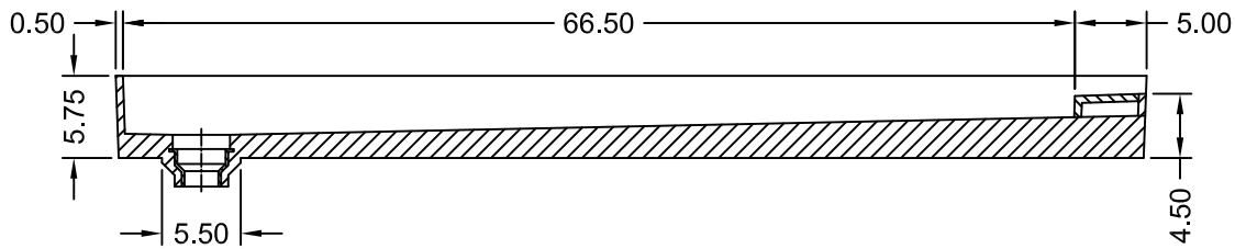
SECTION A-A
