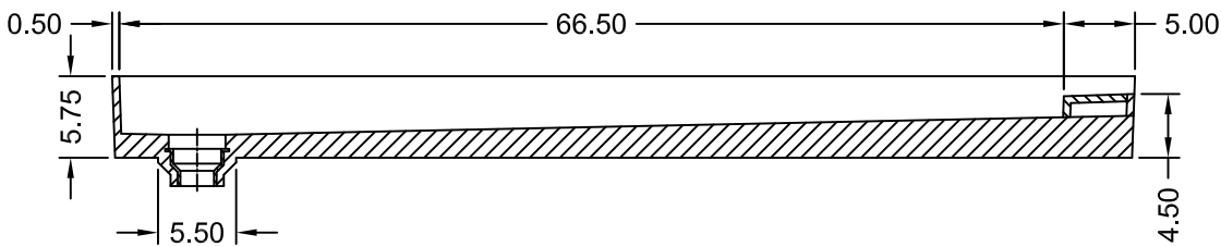
SECTION A-A
