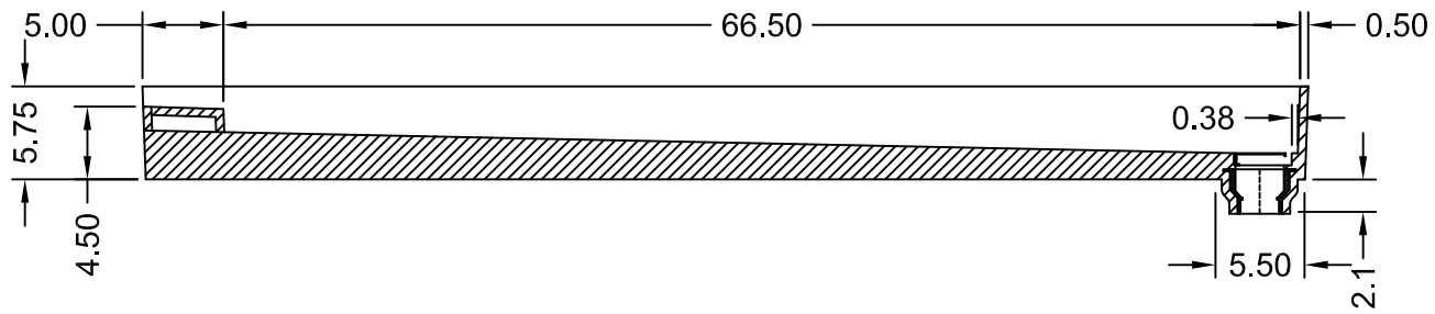
SECTION A-A
