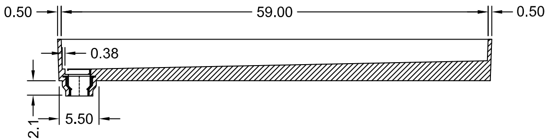
SECTION A-A
